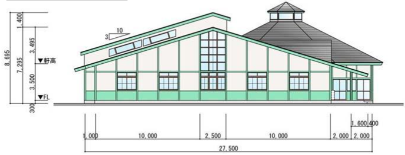
西面立面イメージ
