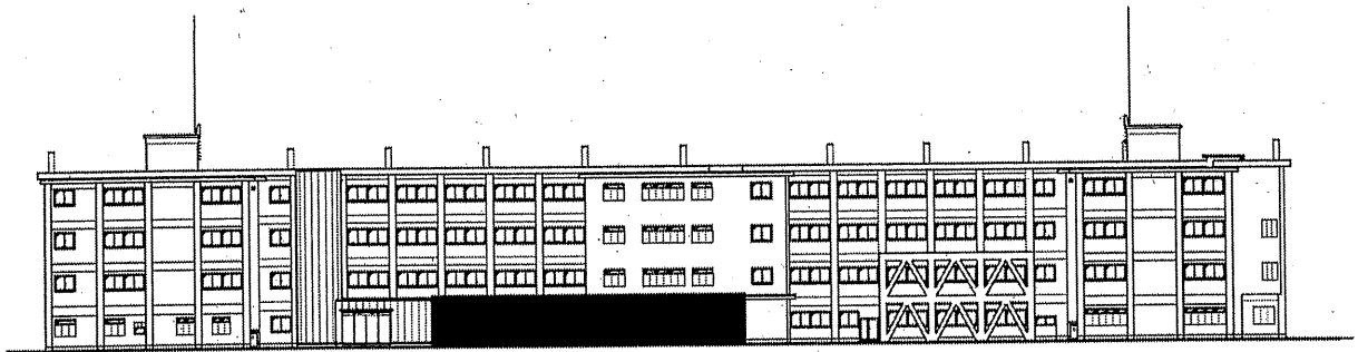
北立面図
