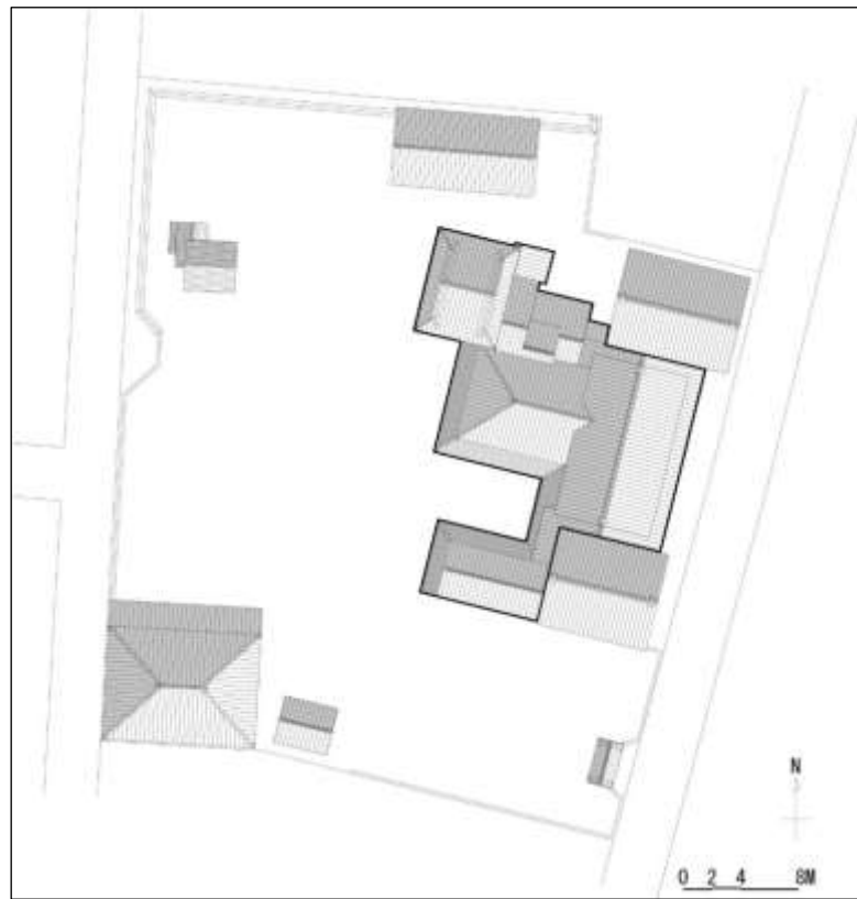
配置図
