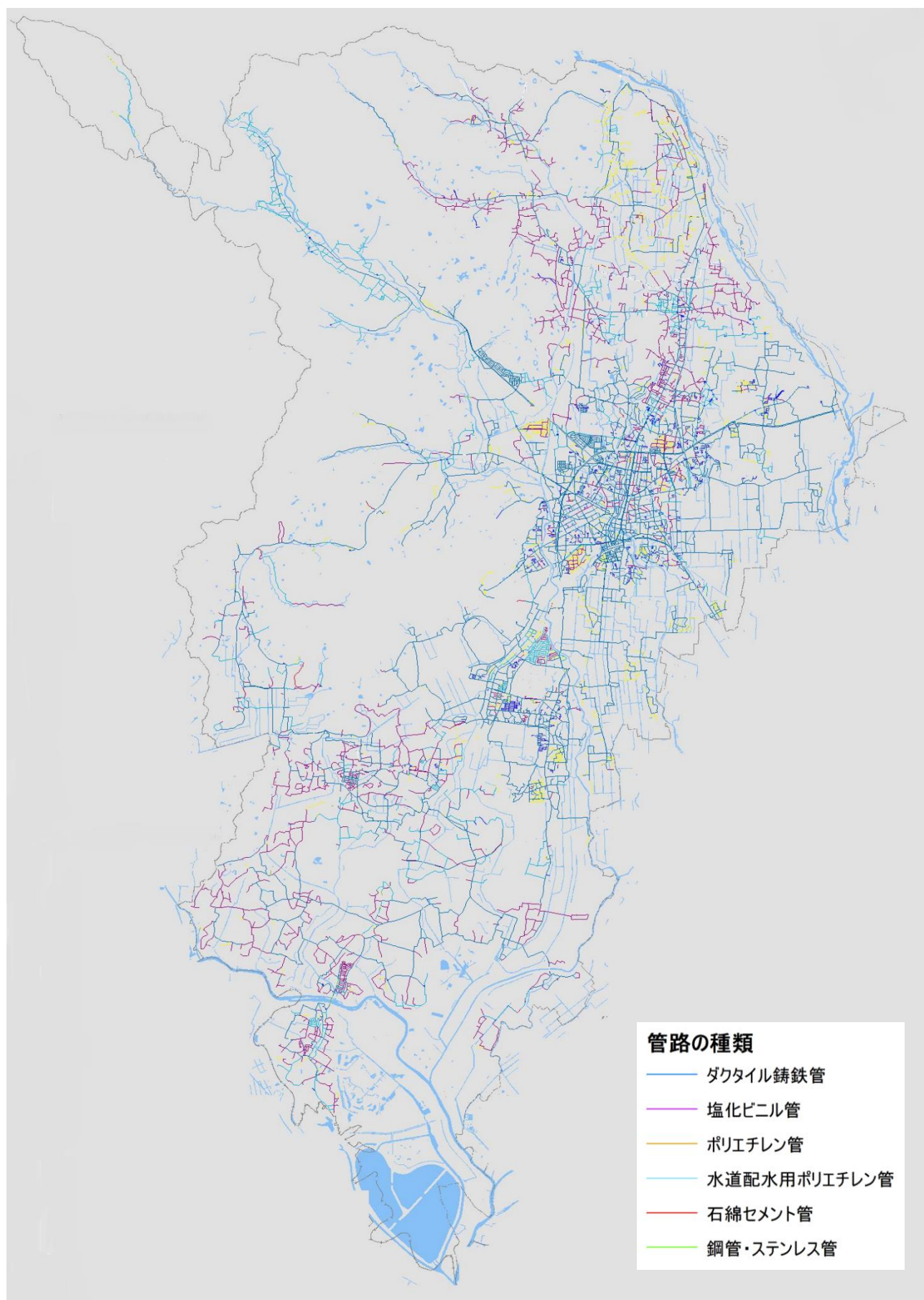
図 2.3 管路の布設状況（令和 4 年度）
