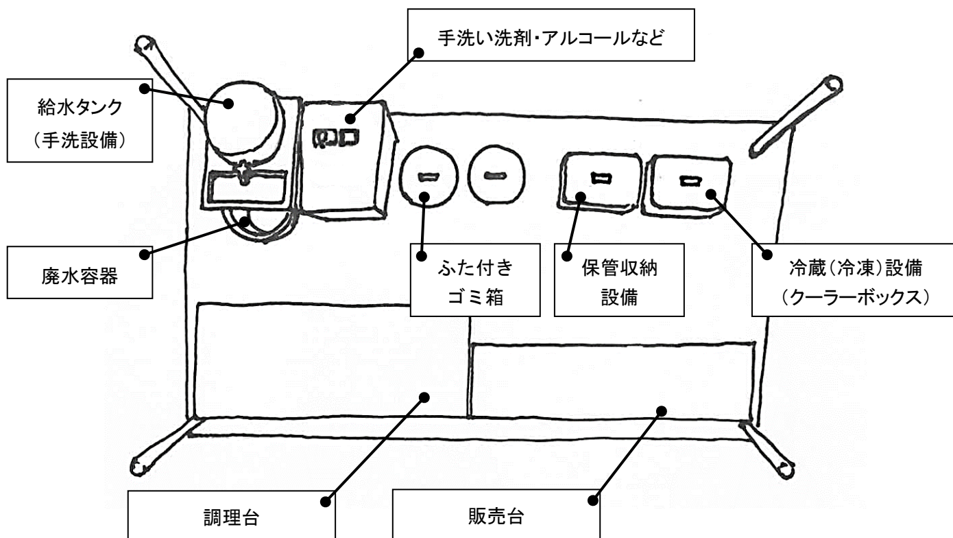
【平面図】
