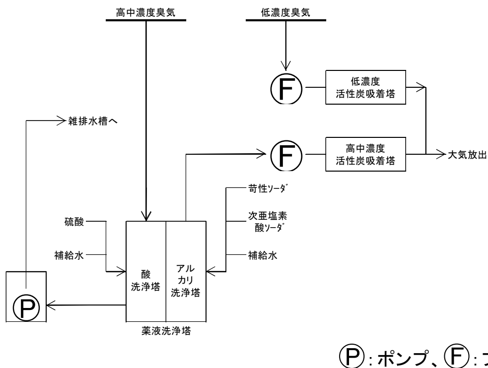
図3-11 処理工程図（脱臭処理）
