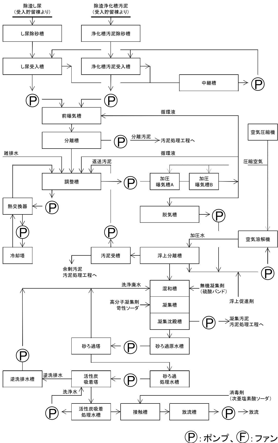
図3-9 処理工程図（水処理棟）
