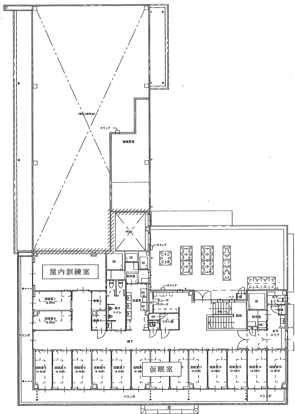
2階平面図
