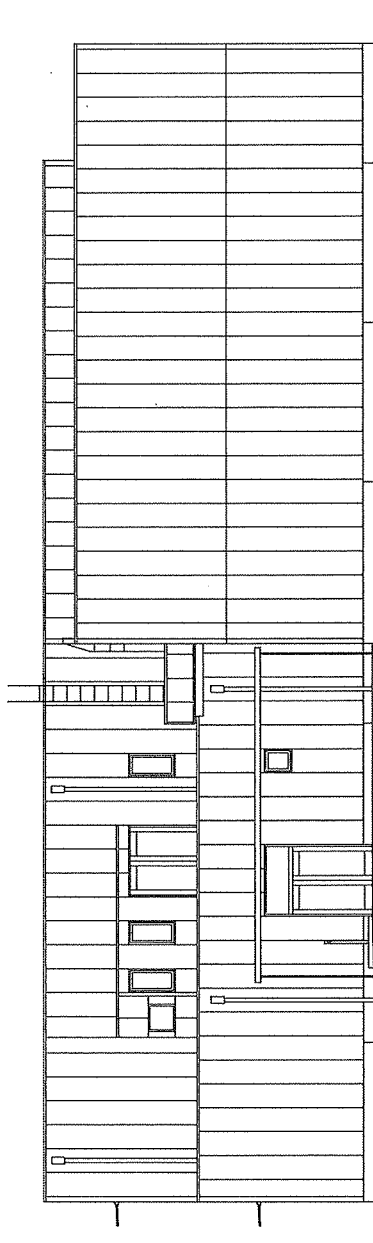
北立面图
