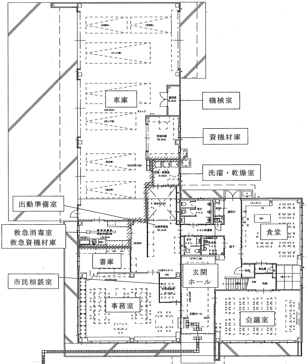
1階平面図
