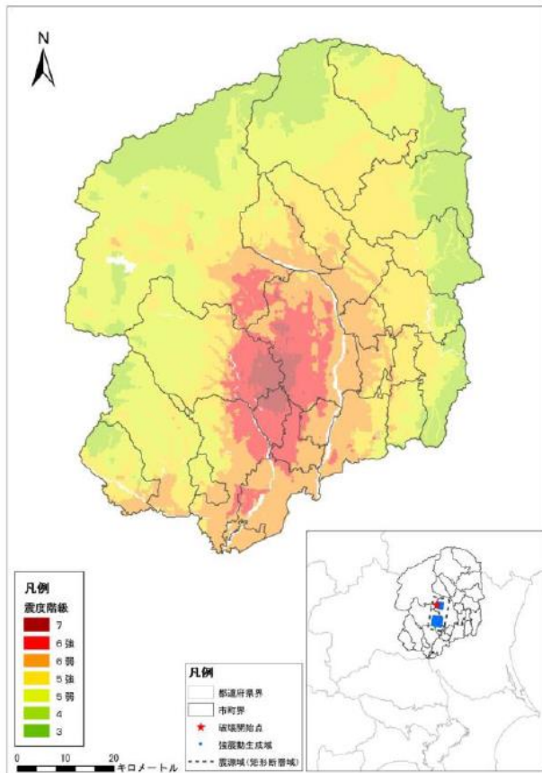
震度分布図 （栃木県庁直下に震源を仮定した地震）
