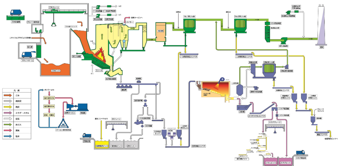
図 1.10 とちぎグリーンプラザ ごみ焼却施設フロー図
